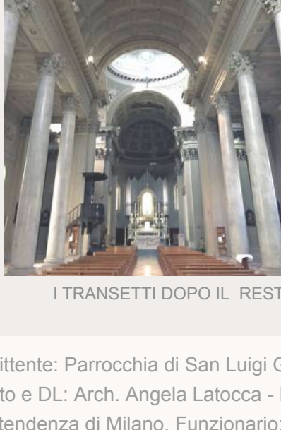
I TRANSETTI DOPO IL RESTAURO DELLA TRABEAZIONE E DELLE VOLTE
